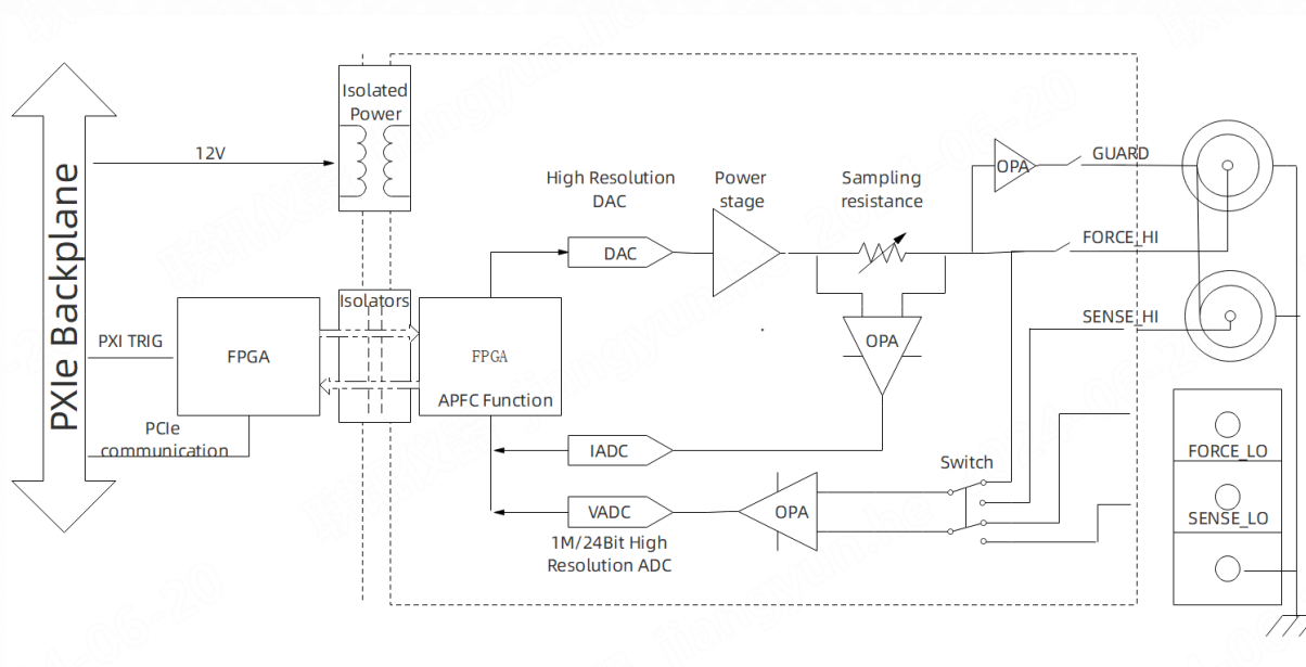
S2016C 架构图
