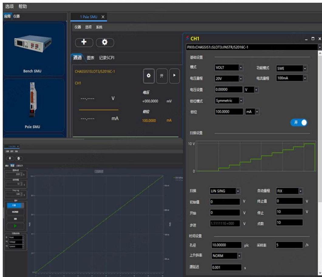
GUI 界面
